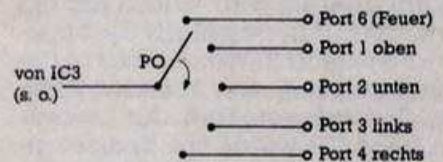
Bild 5. Funktionen-Umschalter
